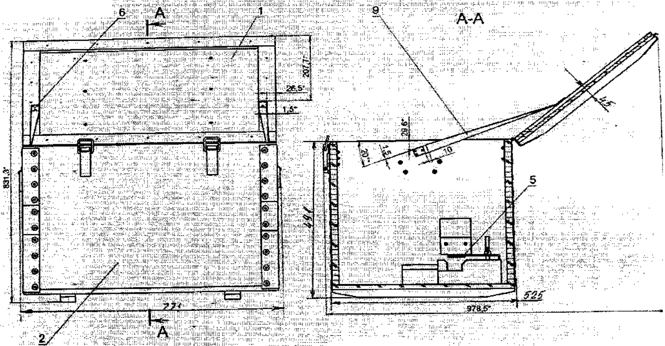
9Պ135 արձակման կայանքի պահպանման և տեղափոխման արկղի հատակի կահավորվածությունը
